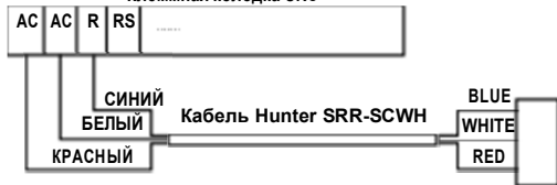
Клеммная колодка SRC
